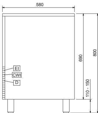
Zij aanzicht
